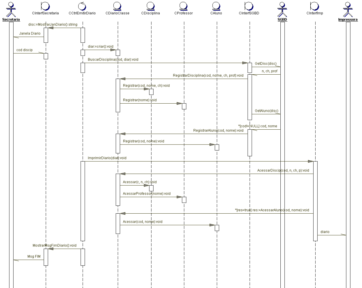
Figura III.16 – Diagrama de seqüência do caso de uso Emitir Diário de Classe.
