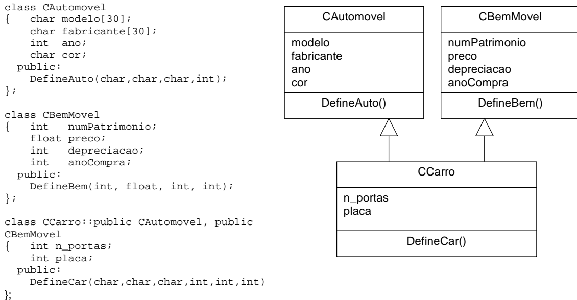
Figura IV.11 – Exemplo de herança múltipla.
