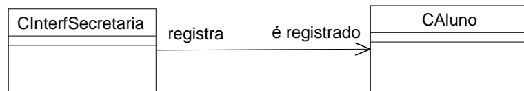
Figura IV.2 – Notação básica para relacionamentos de associação.
