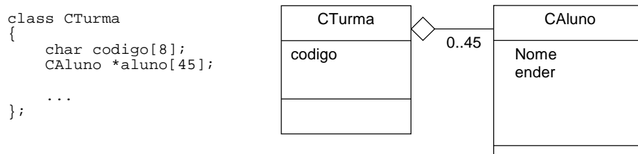
Figura IV.9 – Exemplo de agregação por associação.
