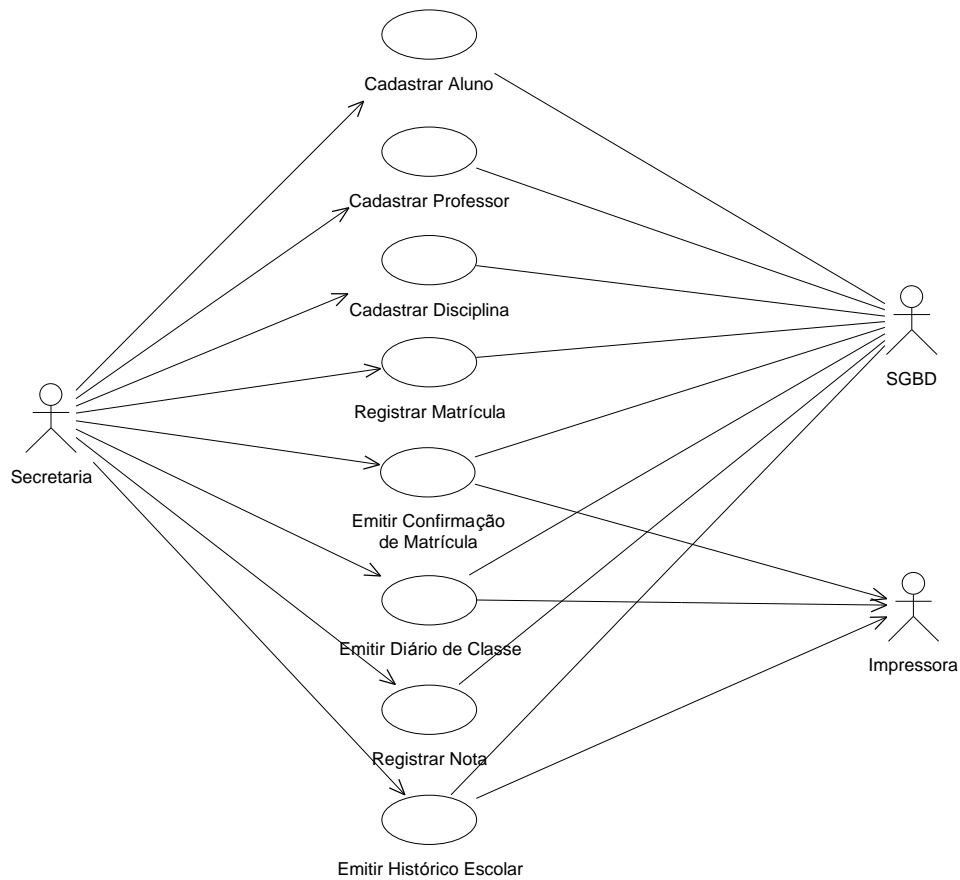
Figura 1.10 – Relacionamentos entre Atores e Casos de Uso.
