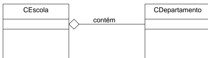
Figura IV.5 – Notação para agregações.
