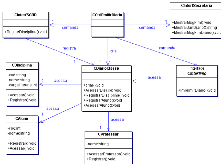
Figura IV.4 – Levantamento de Associações.
