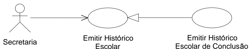
Figura 1.6 – Exemplo de Relacionamento de Generalização entre Casos de Uso
