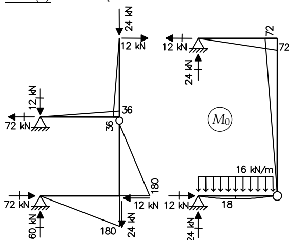
Caso (0) – Solicitação externa isolada no SP
