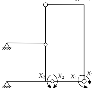
Sistema Principal e Hiperestáticos ( g = 2 )
