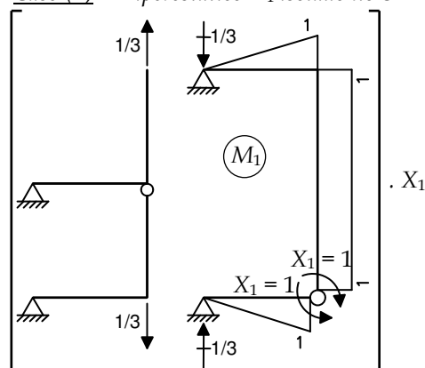
Caso (1) – Hiperestático X_1 isolado no SP
