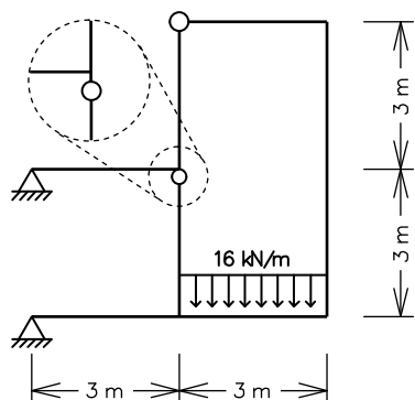
Sistema Principal e Hiperestáticos ( g = 2 )
